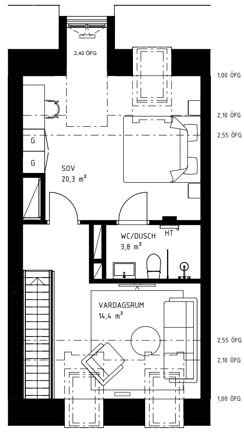
PLAN 2 AV 2, 40,8 KVM Högsta rumshöjd 2,55m
